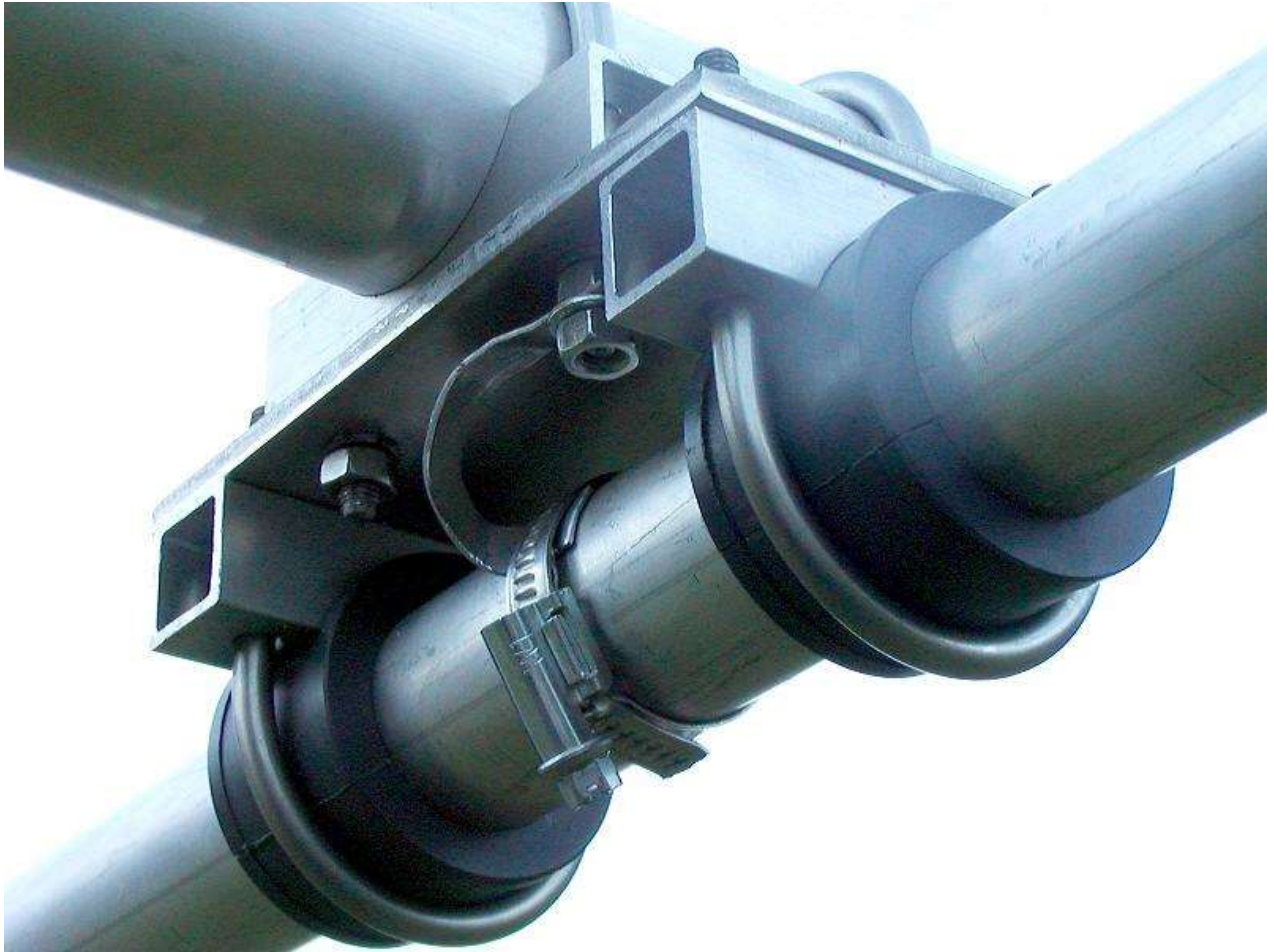
Element bierny polaczony z masa
