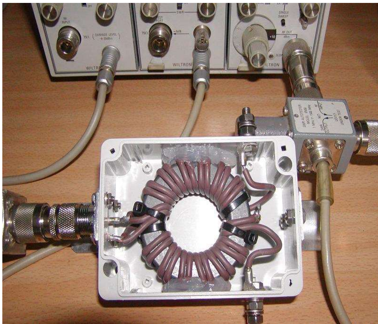
Transformator 4:1 symetryzujący, wykonany na rdzeniu firmy Amidon, wielkość FT-240 (60mm), nawinięty drutem w izolacji teflonowej w opakowaniu odpornym na UV.
