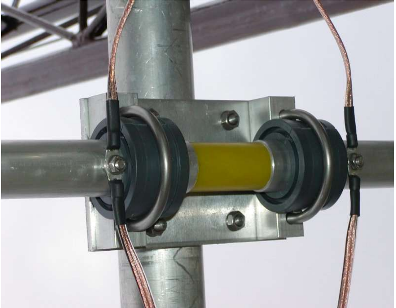
Element czynny + kable fazujące
